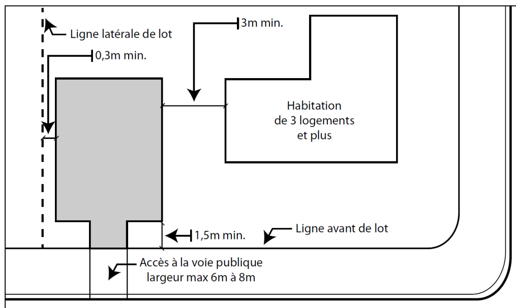
Figure 4 – Exemple d’implantation d’une aire de stationnement pour une habitation de trois logements et plus
